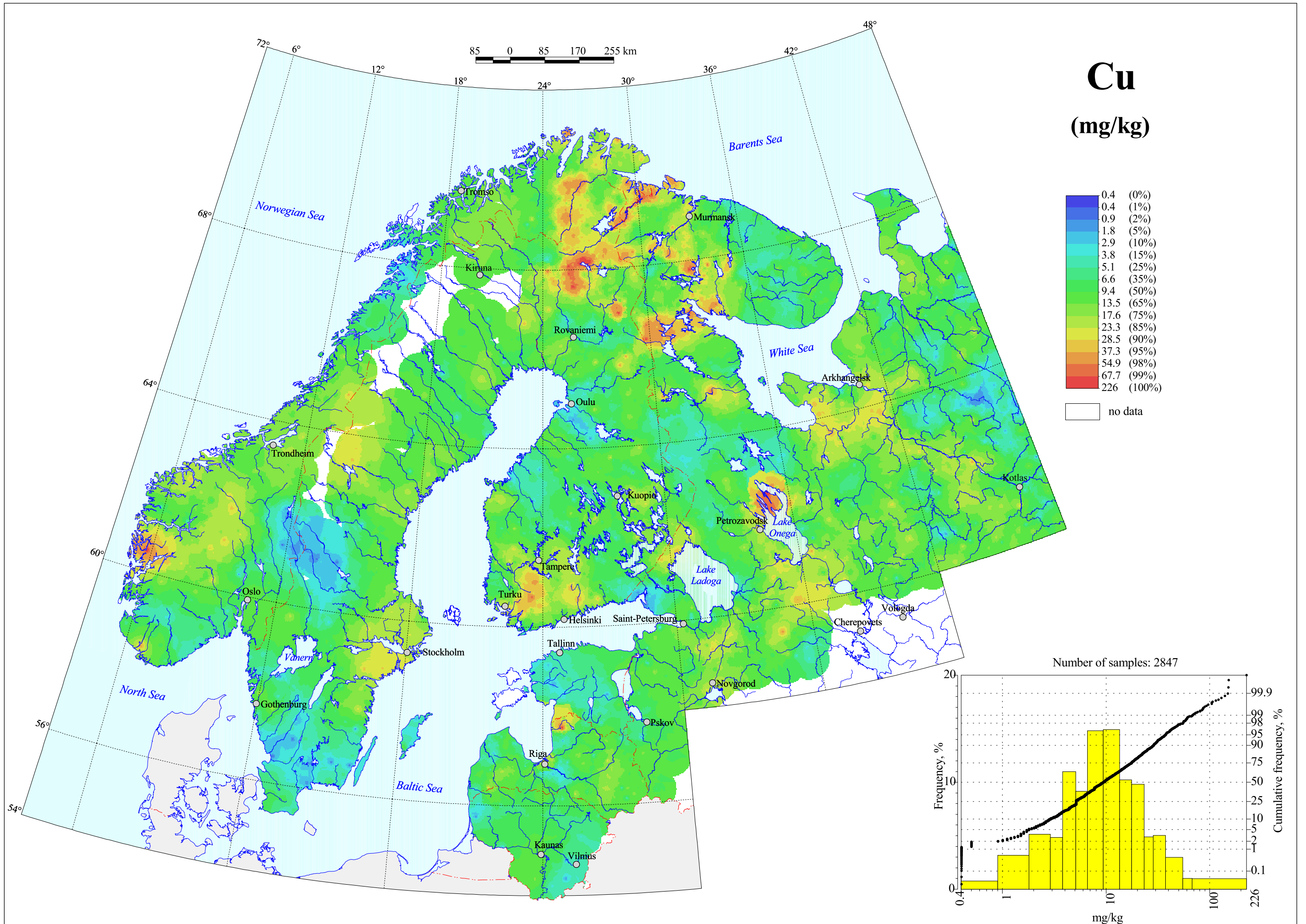
Copper in C-horizon, Grain Size <2 mm, Aqua regia Extraction
